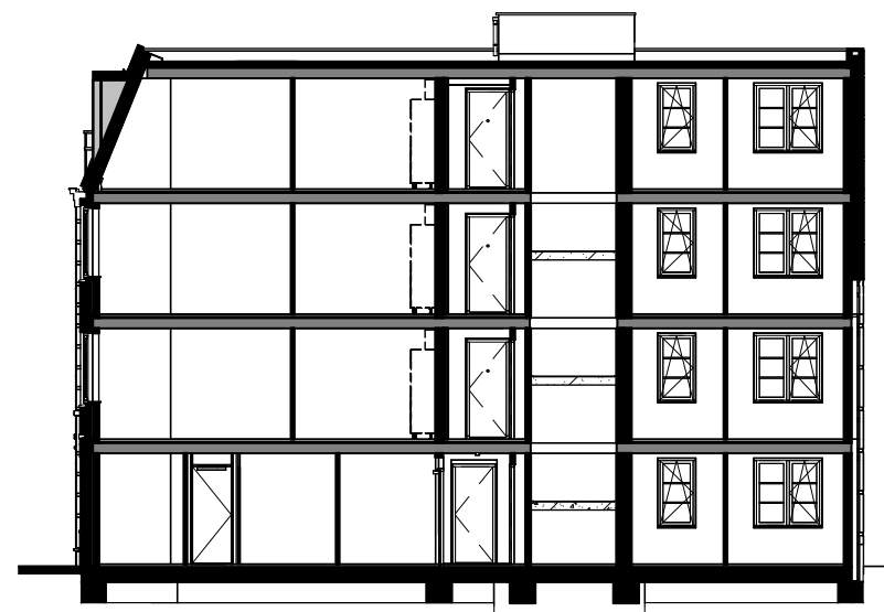
doorsnede B3
